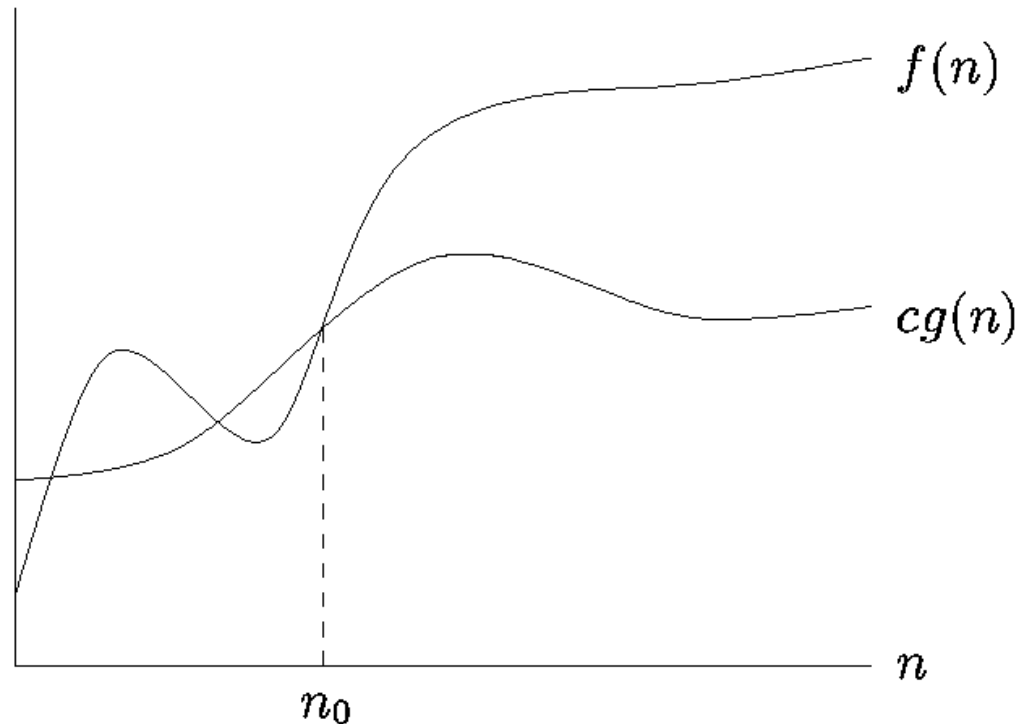
Σχήμα 2.4: f = \Omega(g)
